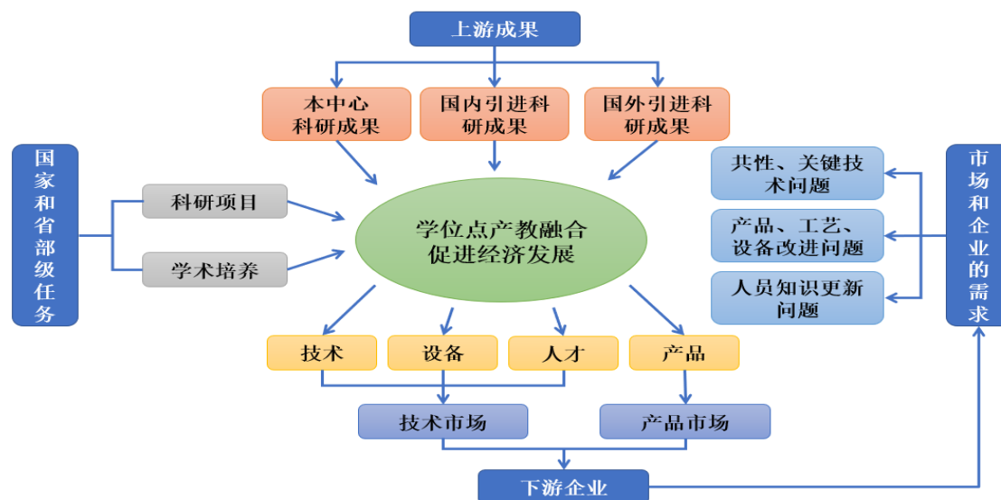
图 3 服务经济发展运行机制
